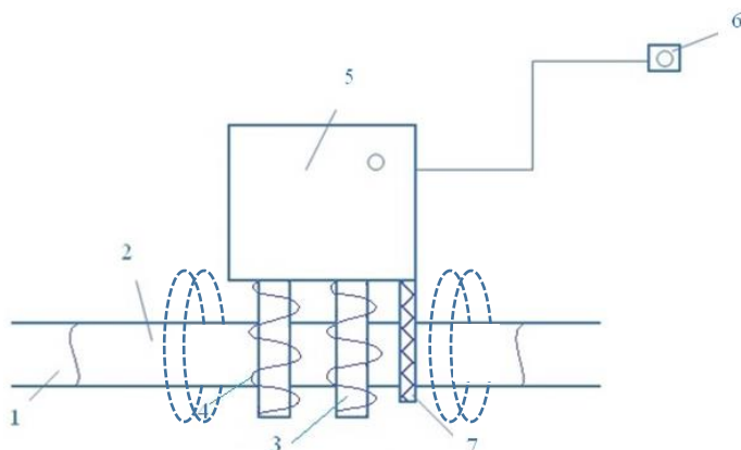
Рис. 3. Устройство для предотвращения образования накипи
