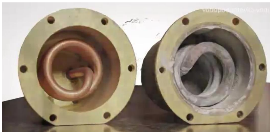
Рис. 1. Фотография теплообменных поверхностей с накипью и без
