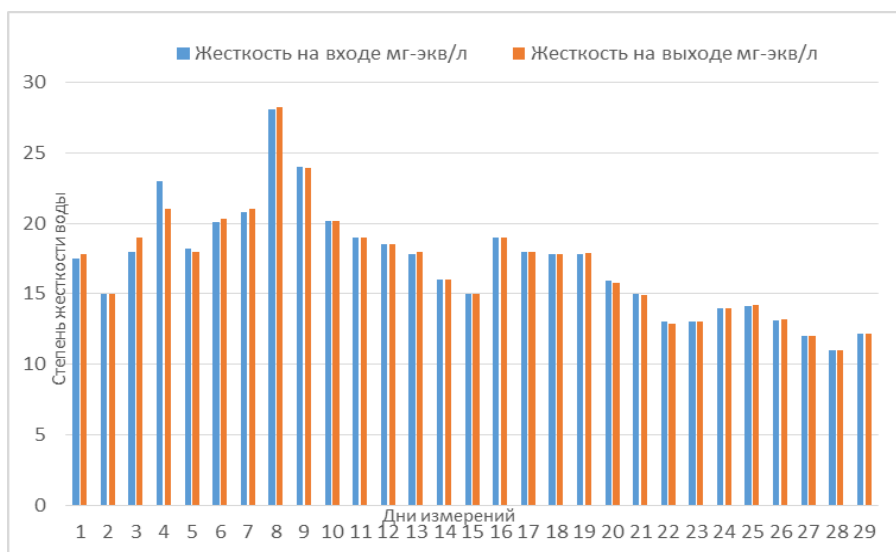
Рис. 4. Диаграмма изменения жесткости обрабатываемой воды
